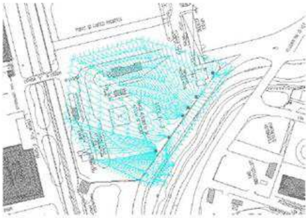
Schema costruttivo punti di estrazione - non in scala
