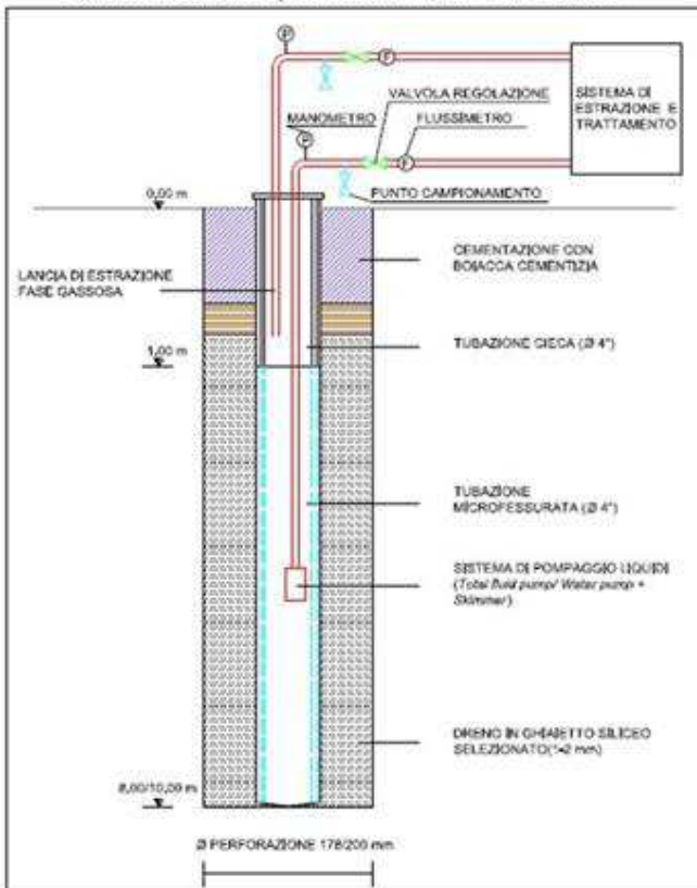
Schema costruttivo punti di estrazione - non in scala
